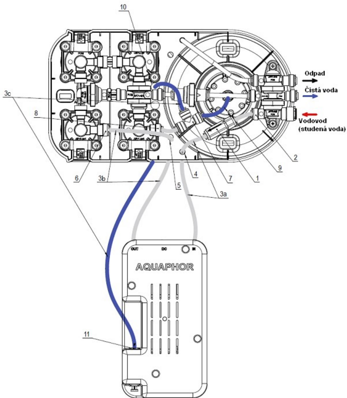
Obr. 6. Schéma připojení KPD vedení 1 k automatu na pitnou vodu Aquaphor Morion DWM-101
