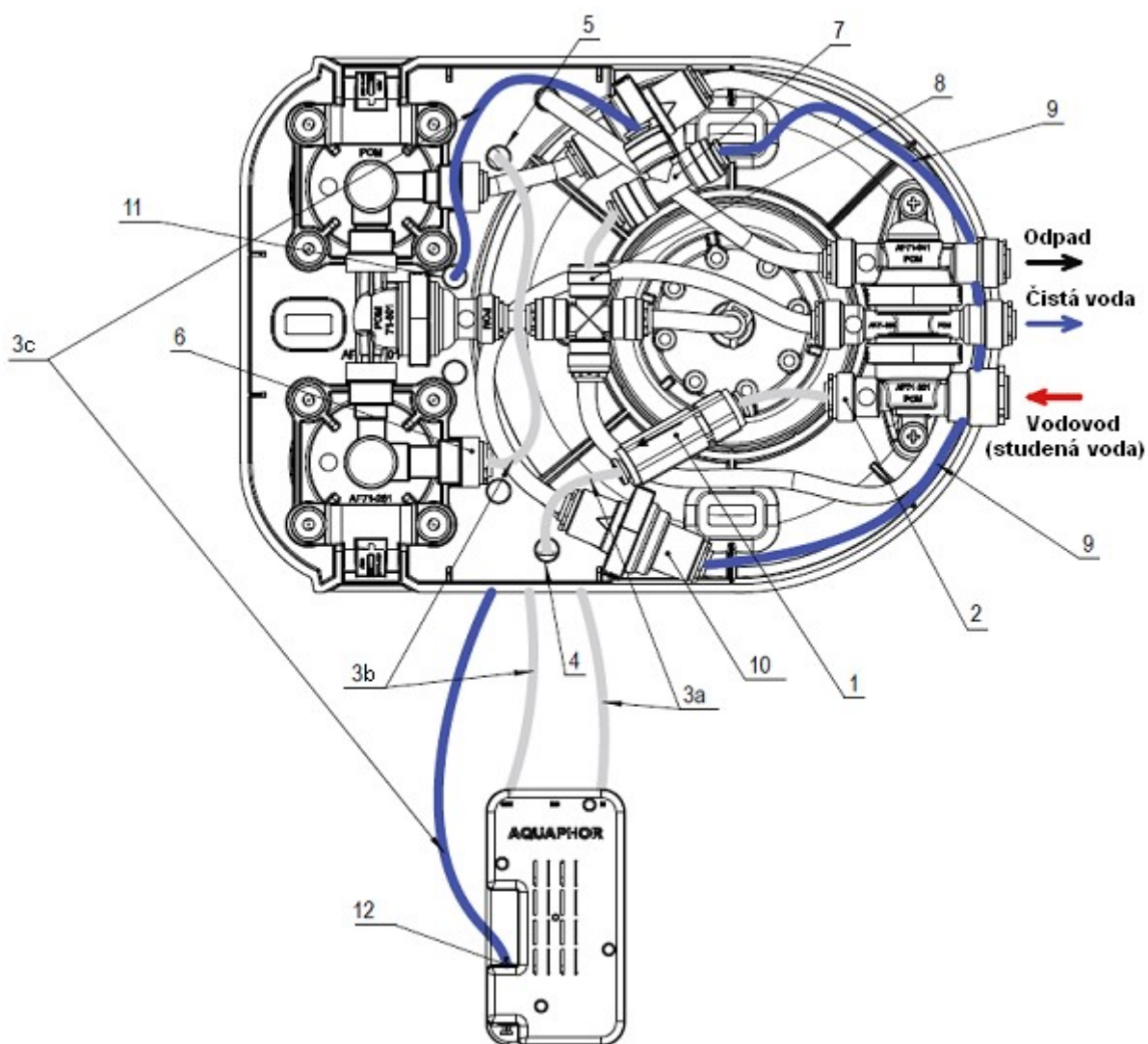
Obr. 7. Schéma připojení KPD vedení 1 k automatu na pitnou vodu Aquaphor DWM-70
